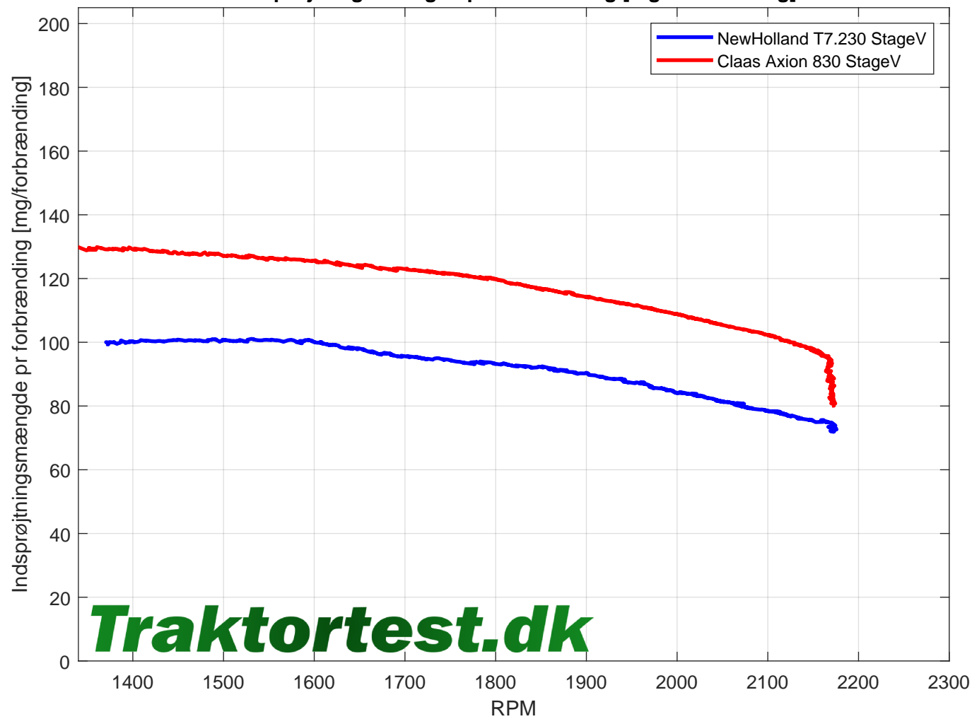
Indsprøjtningmængde pr forbrænding [mg/forbrænding]
