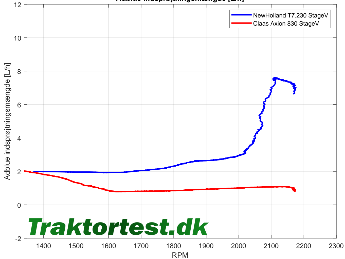
Adblue indsprøjtningmængde [L/h]
