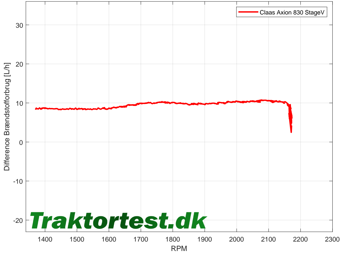
Difference Brændstofforbrug [L/h]
