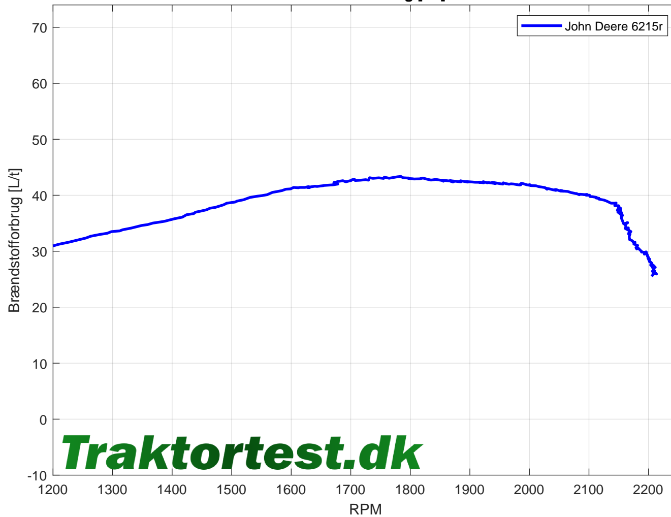
Brændstofforbrug [L/t]
