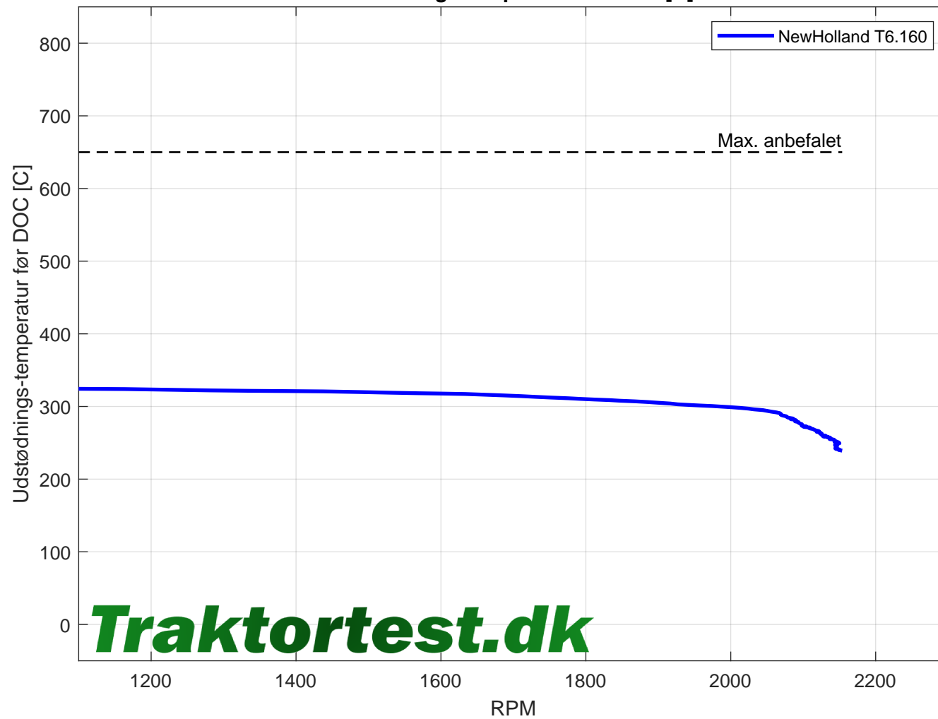
Udstødnings-temperatur før DOC [C]
